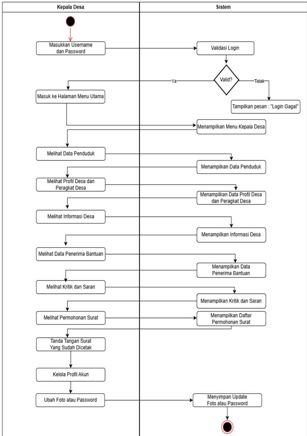
Gambar IV. 3 Activity Diagram Kepala Desa
