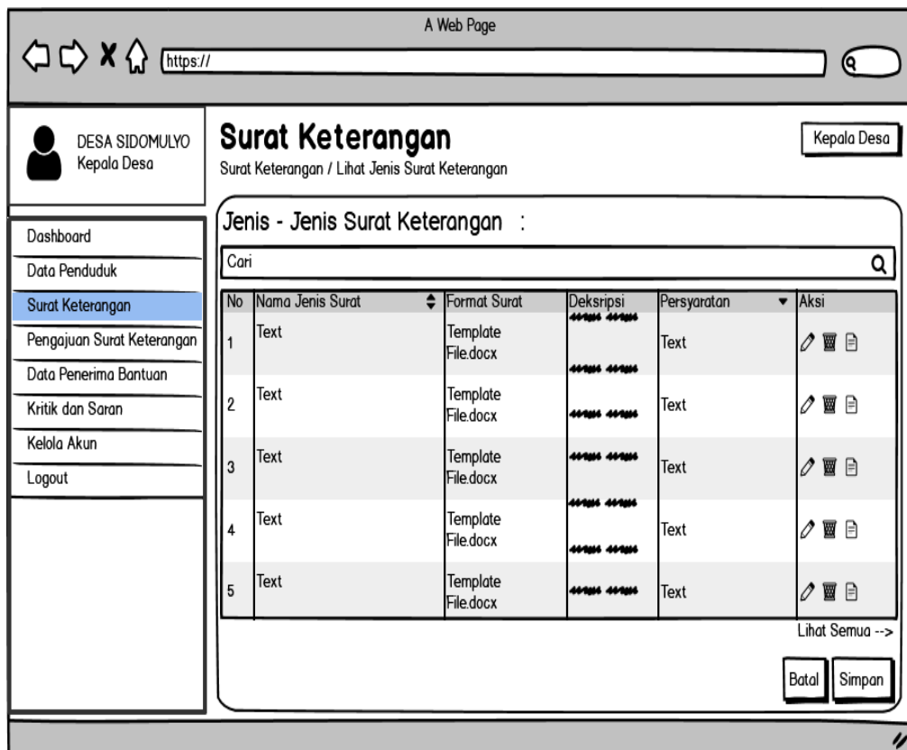
Gambar IV. 30 Halaman Surat Keterangan
