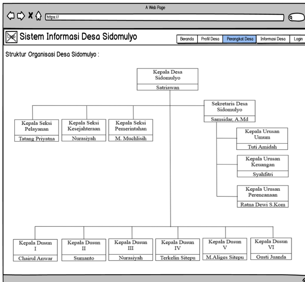
Gambar IV. 8 Halaman Perangkat Desa (Publik)
