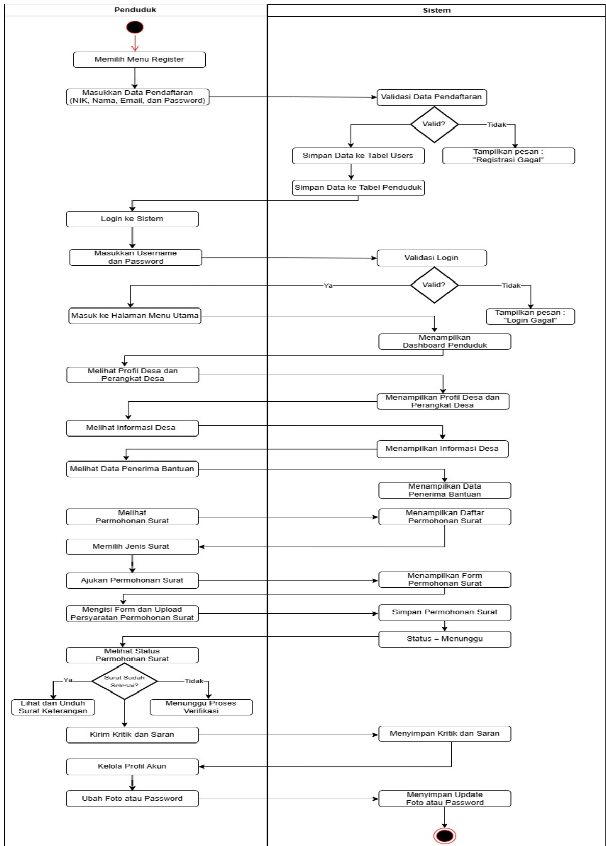
Gambar IV. 4 Activity Diagram Penduduk
