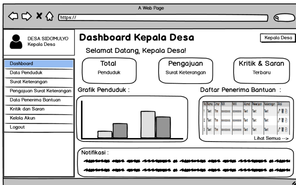
Gambar IV. 28 Halaman Dashboard (Kepala Desa)
